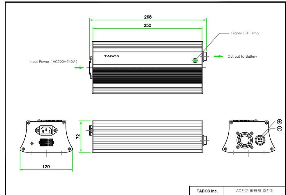
충전기 외곽도(기본형) ( 2015.10.28 )
