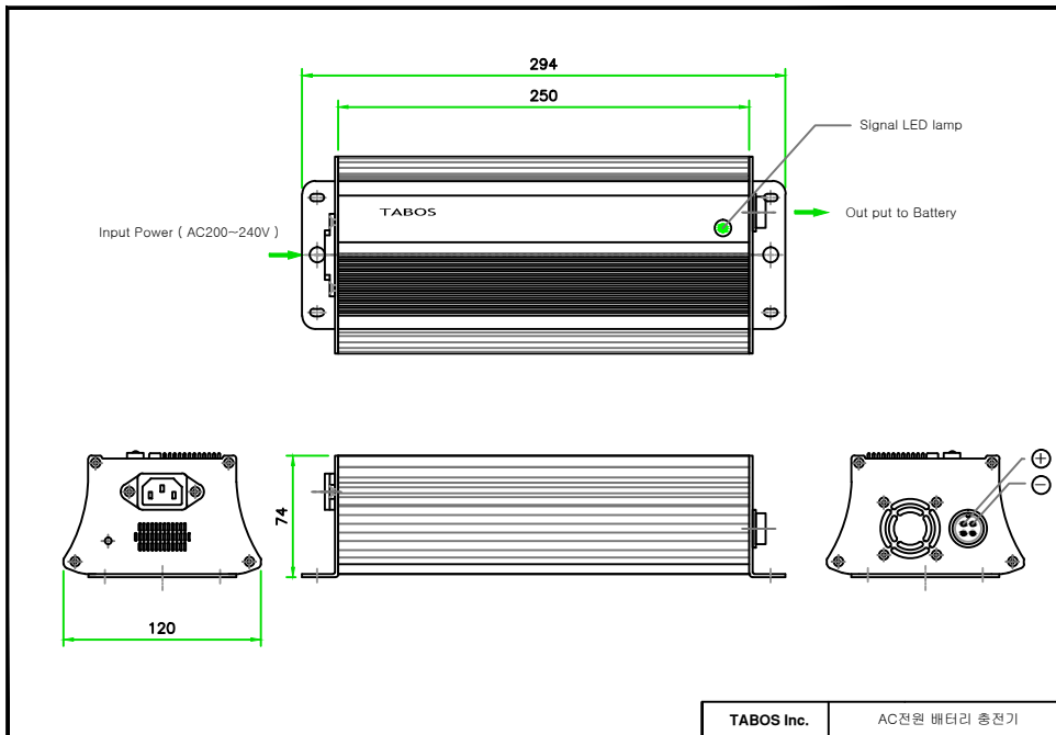
충전기 외곽도(L형) ( 2015.10.28 )
